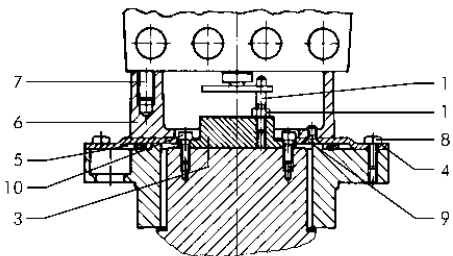
Bild 4.2 · Antrieb 320 cm 2
