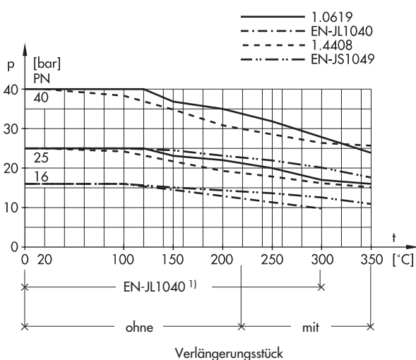
Bild 3 · Druck-Temperatur-Diagramm
