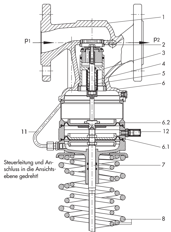
SAV Typ 44-9 (DN 40), Flanschgehäuse
