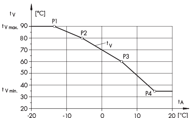
Bild 6 · Vier-Punkte-Kennlinie
