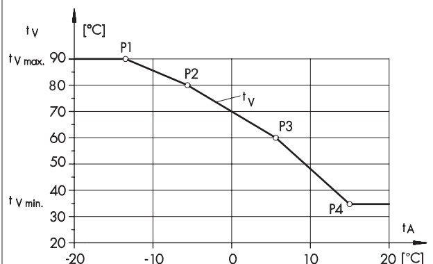
Bild 6 · Vier-Punkte-Kennlinie
