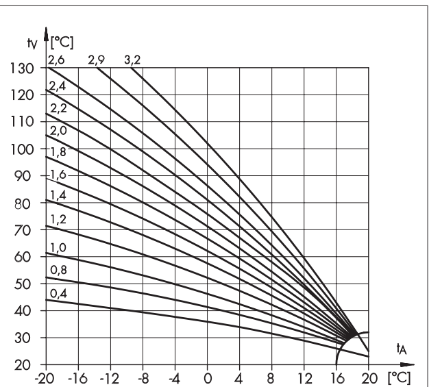
Bild 4 · Heizkennlinie
