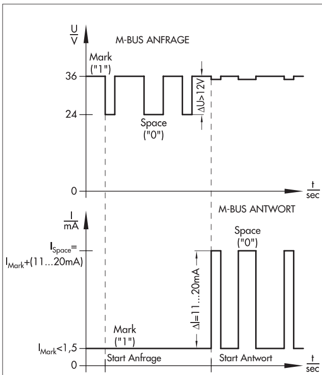
Bild 2 · MASTER SLAVE, Spannungs-/Strom-Pulsdiagramm Anfrage von Master: Wechsel von 36 V (H = "1") auf 24 V (L = "0") Antwort adressierte Slave: bitweises Umschalten des Ruhestroms von 1,5 mA (H = "1") auf ca. I_{\text{Mark}} (1,5 mA) + 11...20 mA (L = "0")
