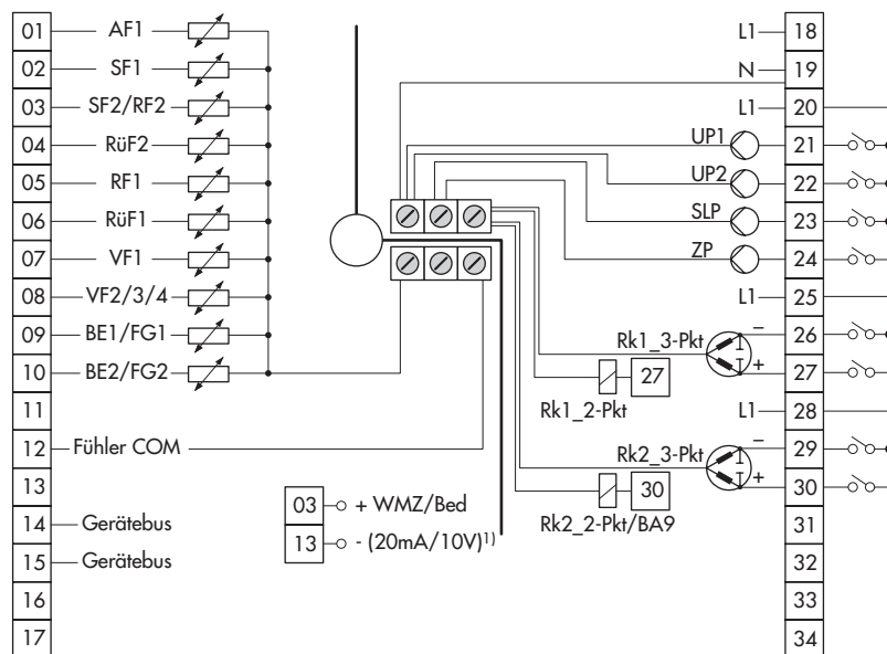
Bild 5 · Anschlussbelegung der Regler TROVIS 5575-000x und TROVIS 5575-002x
