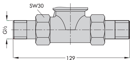
Stellventil mit Anschraubenden
