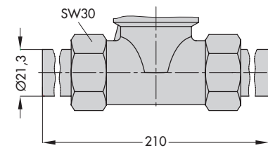
Stellventil mit Anschweißenden
