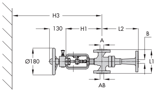
Typ 3267/3273: DN 15 bis 80
