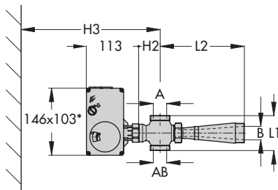
Typ 3267/5824: DN 15 bis 32 Typ 3267/5825: DN 15 bis 32 Typ 3267/5724: DN 15 bis 32 Typ 3267/5725: DN 15 bis 32 * Maße für Typen 5824-13, 5825-13, 5724-13 und 5725-13: 146 x 136
