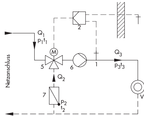
Bild 4 · Vereinfachtes Anlagenwirkbild eines Verbraucherkreislaufs mit Umwälzpumpe und Dreiwegeventil
