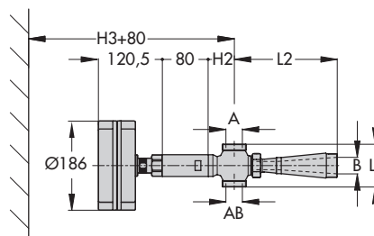
Ausführung mit Isolierzwischenstück für Temperaturen bis 150 °C
