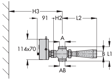
Typ 3267/5857: DN 15 bis 25 Typ 3267/5757: DN 15 bis 25
