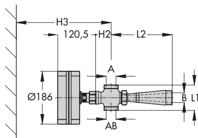
Typ 3267/2780-1: DN 15 bis 32
