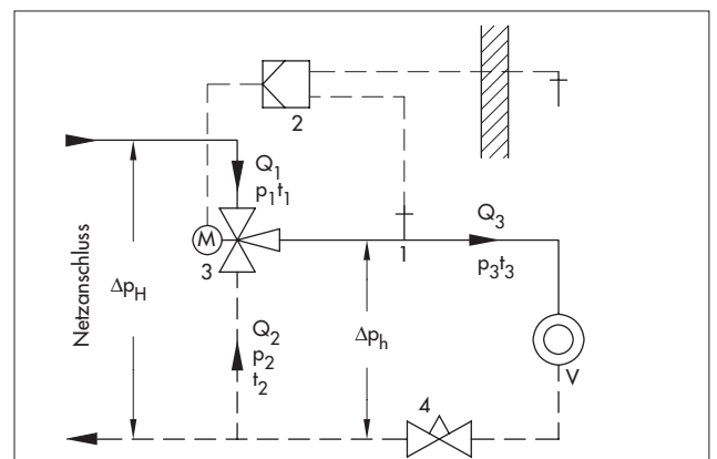
Bild 3 · Vereinfachtes Anlagenwirkbild eines Verbraucherkreislaufs mit Strahlpumpe
