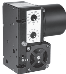
Bild 2 · PI-Reglerbaustein Typ 3434-2
