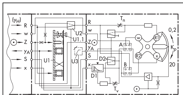
Regler- u. Leitstation Hand-Automatik-Umschalter Typ 3424-45 PID-Reglerbaustein Typ 3423-3
