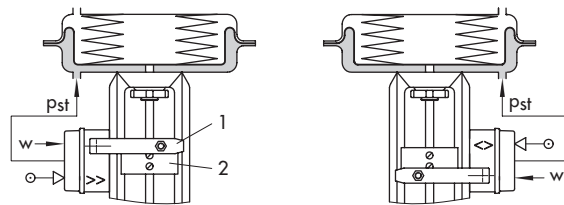
Bild 5: Wirkrichtung >> Anbau links
