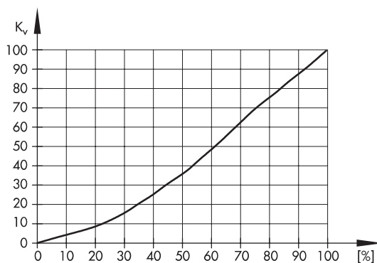
Bild 6 · Natürliche Kennlinie
