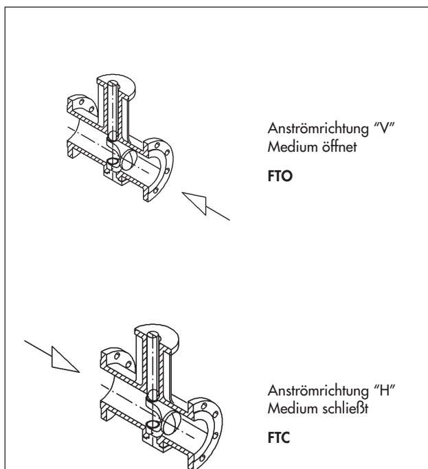
Bild 4 und 5 · Anströmrichtungen V und H
