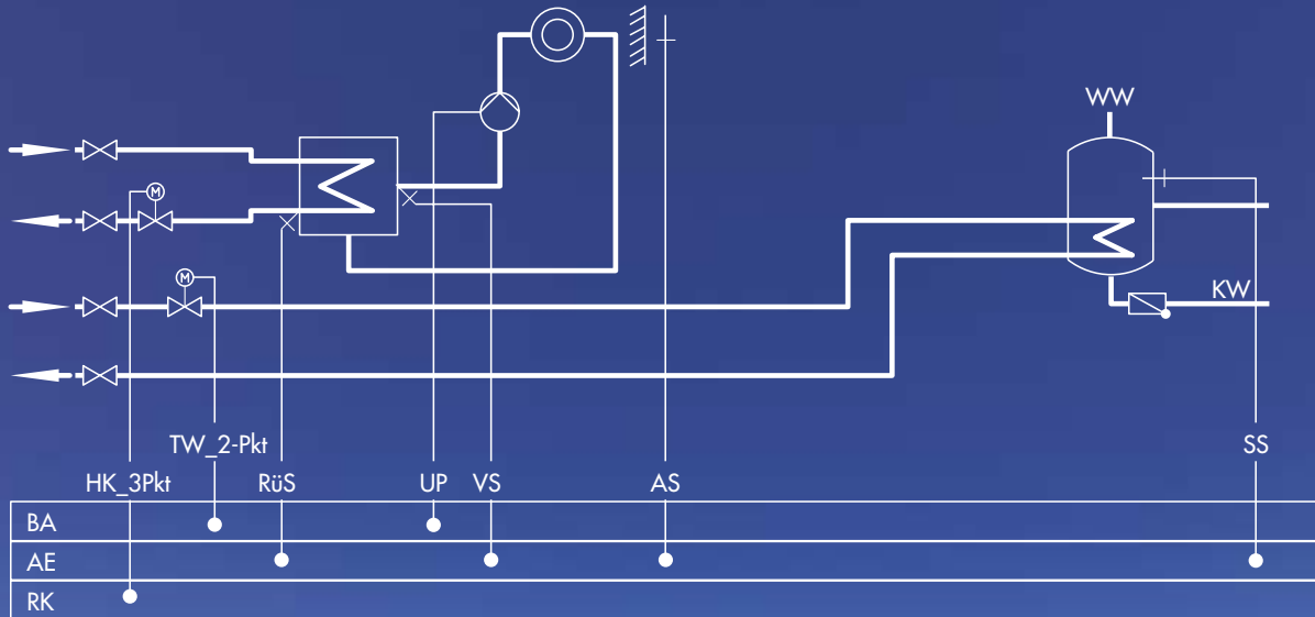
Witterungsgeführter Heizkreis und 2-Punkt-Regelung für primärseitiges Speichersystem mit TROVIS 5432 V2.0
