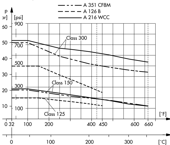
Fig. 4 · Pressure-temperature diagrams
