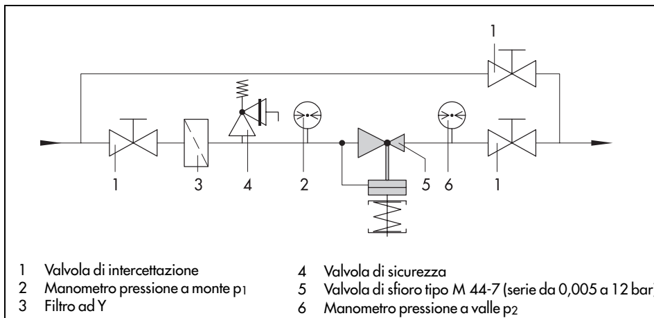
Fig. 3 - Schema d'installazione
