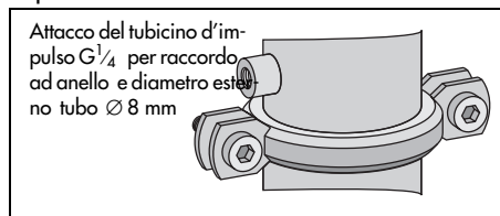
Fig. 4 - Attacco per il tubicino d'impulso G 1/4
