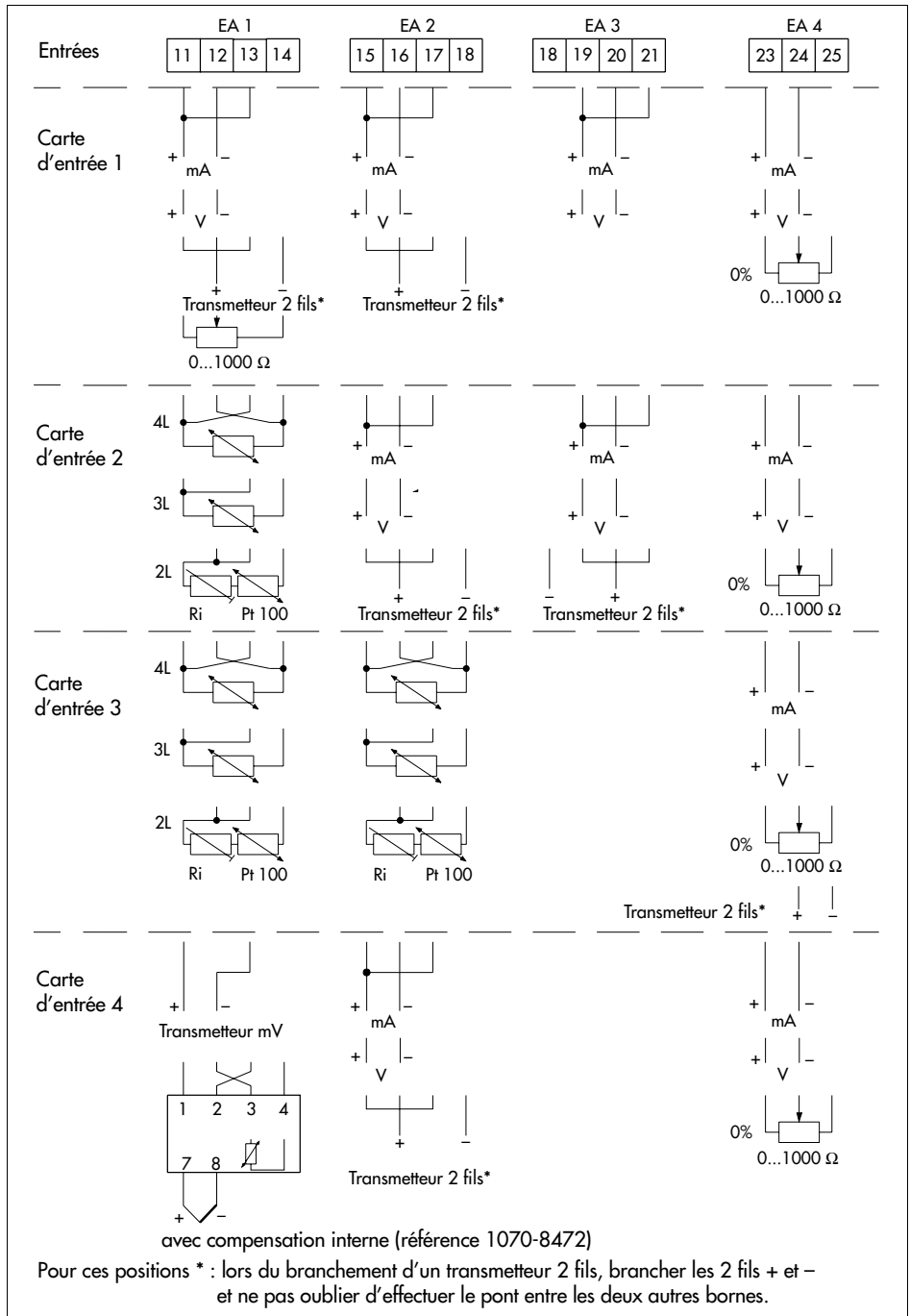
Fig. 8 · Schéma de raccordement TROVIS 6412 (suite)
