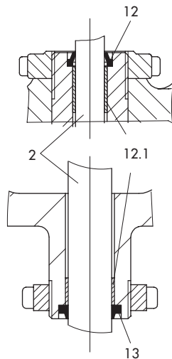
Fig. 6 - Spindel tætning
