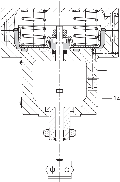
Fig. 3.2 · Type 3277-5 Pneumatisk aktuator for Ventil Serie 240
