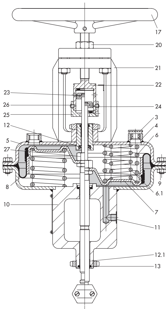
Fig. 5 - Type 3277 Pneumatisk aktuator med håndhjul
