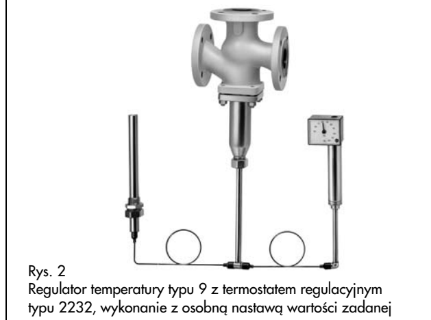
Rys. 2 · Regulator temperatury typu 9 z termostatem regulacyjnym typu 2232, wykonanie z osobną nastawą wartości zadanej
