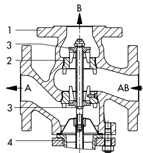
Rys. 4 · Zawór trójdrogowy typu 9 z grzybem w konfiguracji II, strzałki wskazują kierunek przepływu dla pracy w trybie rozdzielającym
