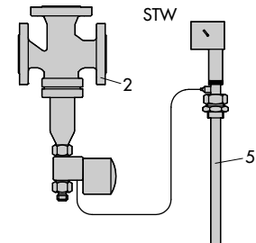
Rys. 7.2 Typ 8/2213 lub typ 9/2213
