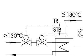
Rys. 4 Instalacja grzewcza zasilana gorącą wodą z regulatorem temperatury i ogranicznikiem temperatury bezpieczeństwa według DIN 4752
