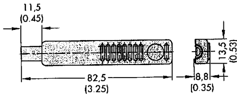
Fig. 8 - Module COPA
