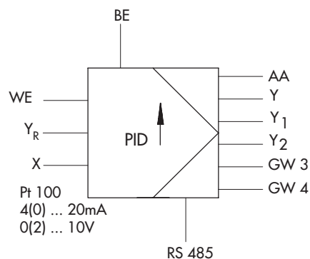
Fig. 3 - TROVIS 6497 con uscita costante
