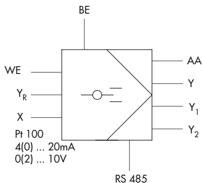
Fig. 2 - TROVIS 6497 con uscita in commutazione
