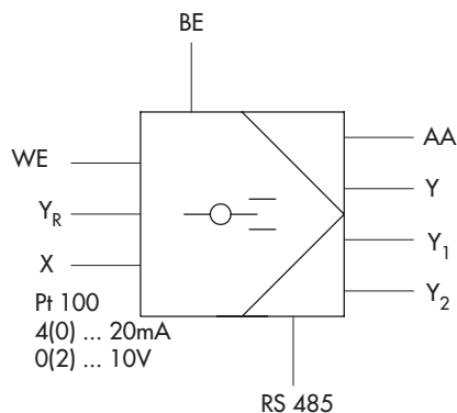
Rys. 2 · TROVIS 6497 z wyjściem sygnałów przełączających
