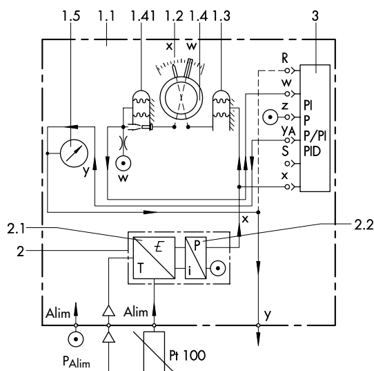
Fig. 4 · Schéma de principe d'un régulateur à consigne interne pour température, exécution avec poste de commande type 3432-01
