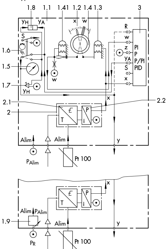
5.1 · Exécution avec poste de réduction d'air (1.9)
