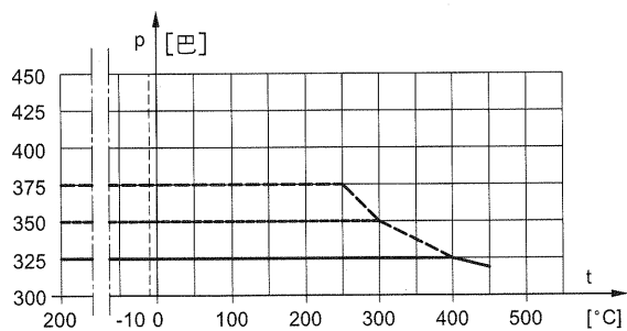
图4·WN1.4571用的压力-温度图表
