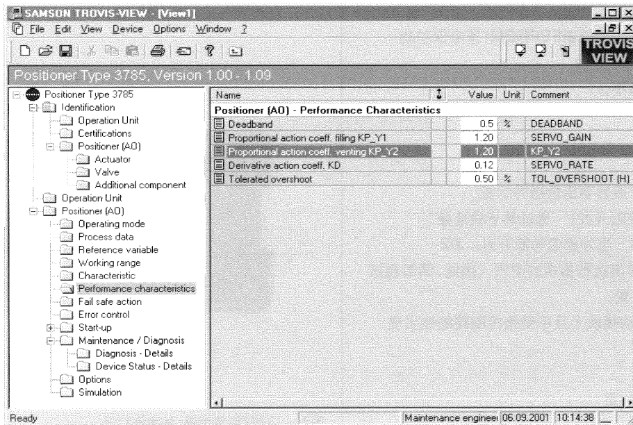
图4 · 使用TROVIS VIEW软件显示参数
