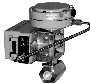
Fig. 2 · Posizionatore Tipo 3730-0 su microvalvola Tipo 3510
