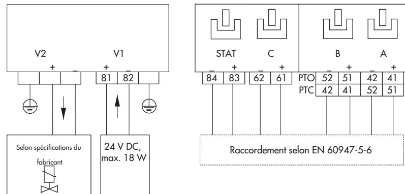
Fig. 6 · Exécution pour électrovanne externe type 3738-20-xxx1000xxx000
