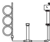
Typ 2235 mit frei verlegbarem Luft- fühler und Schellenbefesti- gung (am Sollwertsteller)
