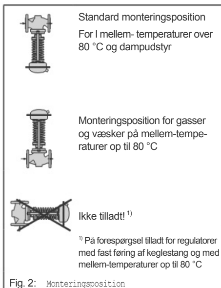
Fig. 2: Monteringsposition
