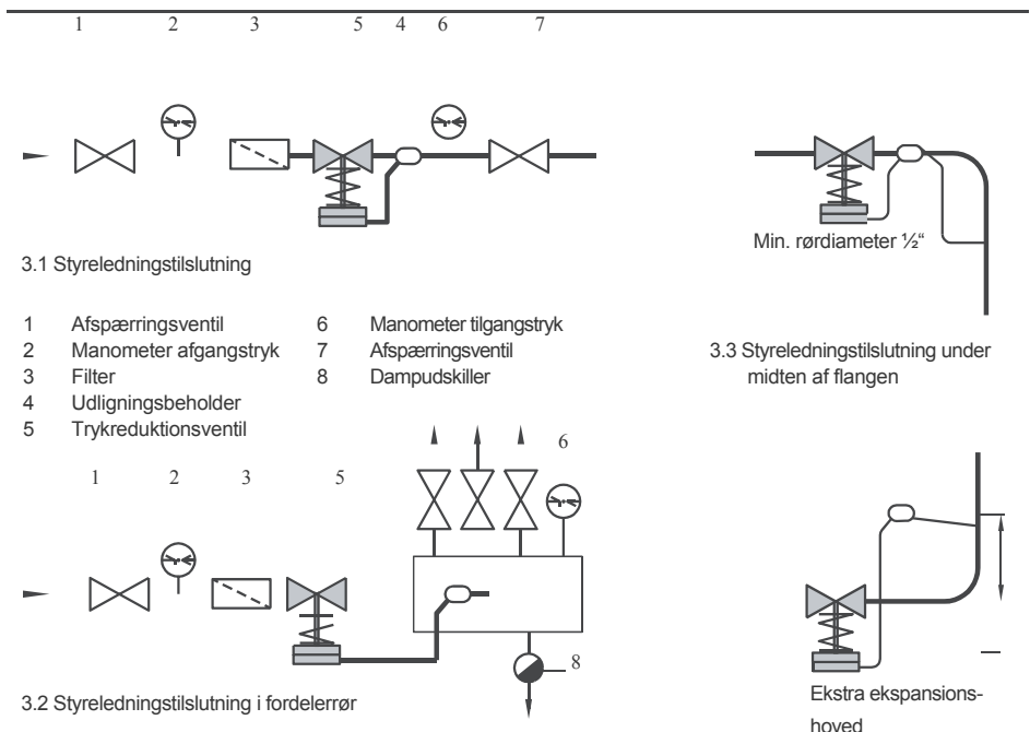
Fig. 3: Eksempler på installation med damp
