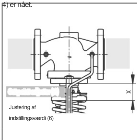
Fig. 4: Justering af indstillingsværdi med dimension x
