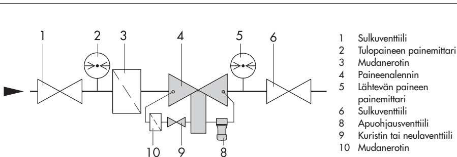
Kuva 3 · Asennusesimerkki
