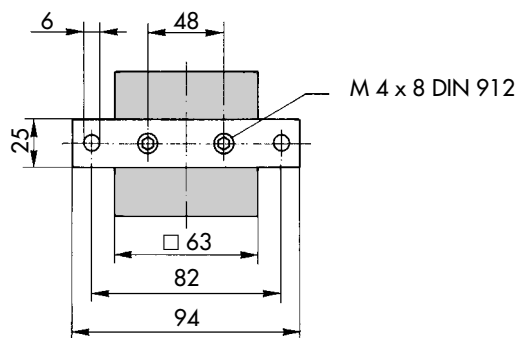
Fig. 2 · afmetingen in mm
