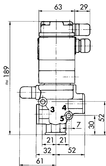
Fig. 3 · afmetingen in mm
