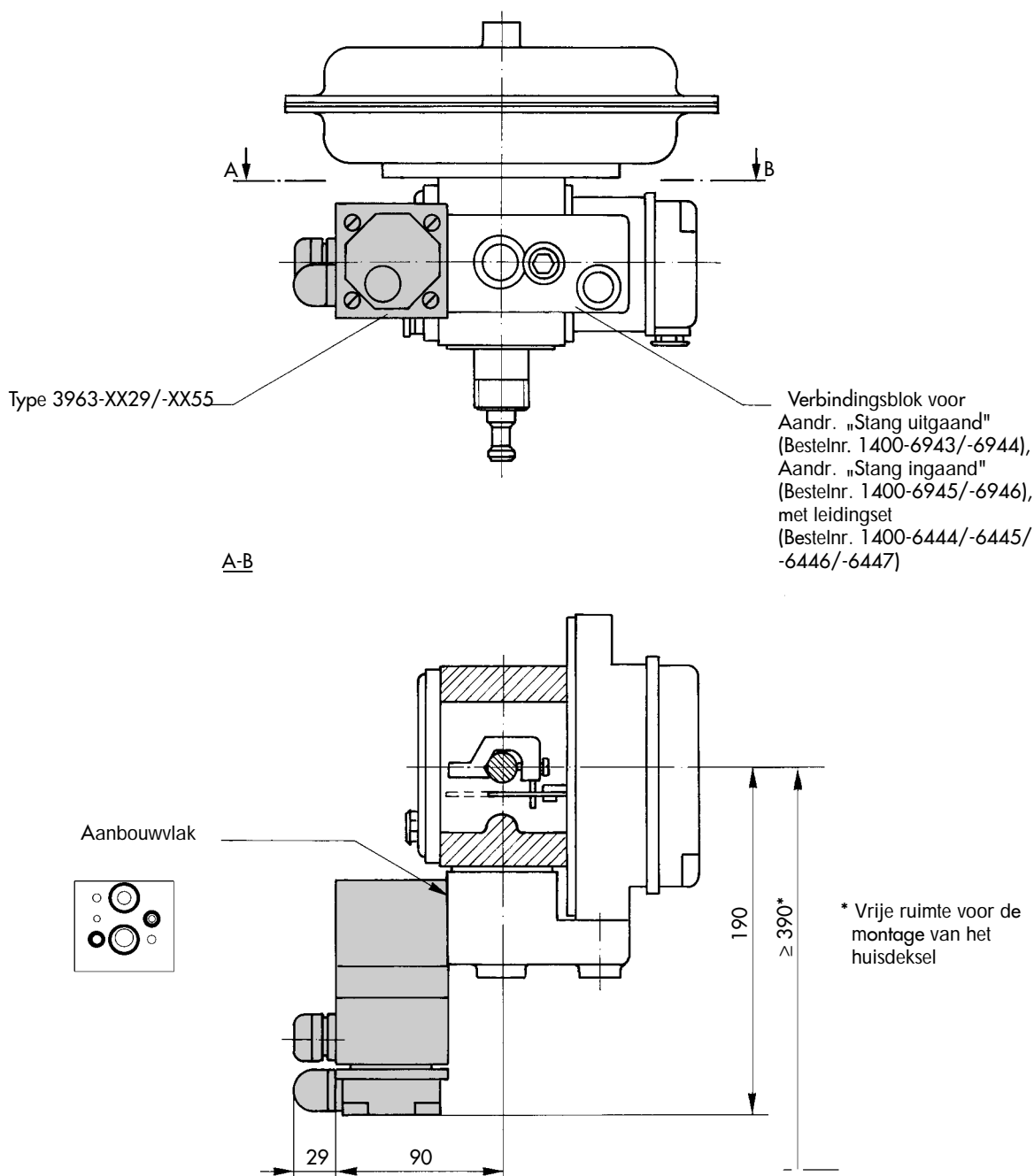
Fig. 8 · afmetingen in mm
