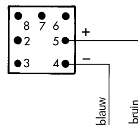
Kabeldoos (fabrikaat Harting)
