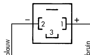
Kabeldoos conform EN 175301-803
