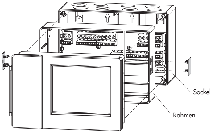
Bild 9 · Wandaufbaumontage
