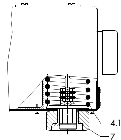
Bild 3 · Typ 5821-5, -6 kraftschlüssig
