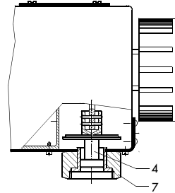
Bild 3 · Typ 5821-5, -6 kraftschlüssig
