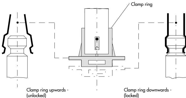
Fig. 7 · Clamp ring
