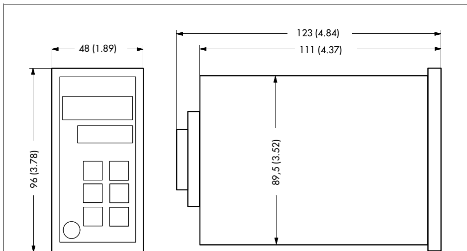
Figura 2 · Dimensiones en mm (inch)
