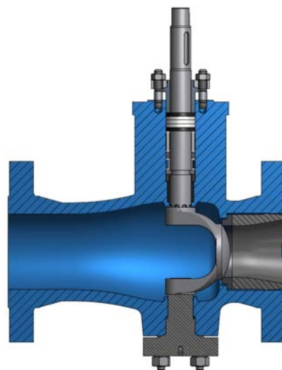
Bild 2: Schnittzeichnung
