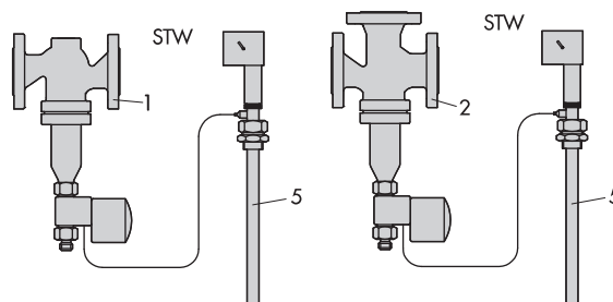
Fig. 7.1 Tipo 2111/2213 o Tipo 2114/2213
