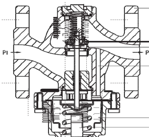
Редукционный клапан Тип 44-1 В · Фланцевое исполнение корпуса из чугуна с шаровидным графитом
