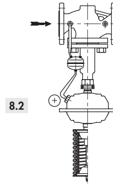
8.2 Aukšto slėgio valdymo linija, aušinimo talpa
