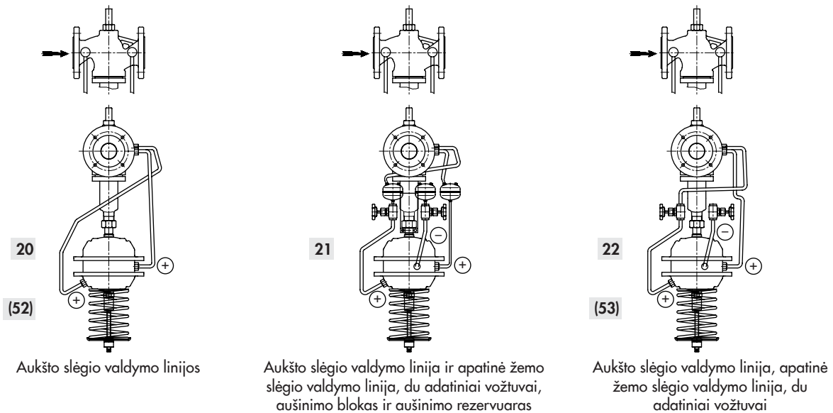
8.7 pav.: Montavimui paruoštos valdymo linijos 42-39 tipai, skirtos montuoti srauto vamzdyje
