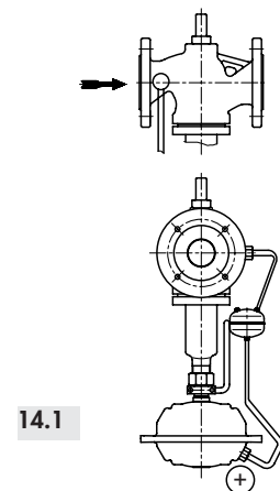
14.1 Aukšto slėgio valdymo linija, aušinimo rezervuaras su laikikliu tvirtinimui
