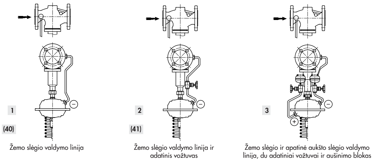
8.1 pav.: Montavimui paruoštos valdymo linijos 42-24 tipui ir 42-28 tipui, skirtos montavimui grįžtamojo srauto vamzdyje
