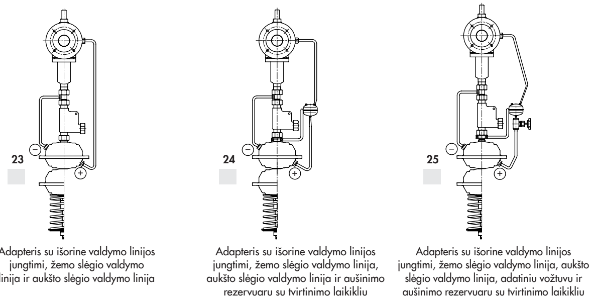
8.8 pav.: Montavimui paruoštos valdymo linijos 42-36 DoT tipai ir 42-37 DoT tipai
