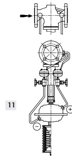
11 Žemo slėgio ir aukšto slėgio valdymo linija, du adatiniai vožtuvai ir aušinimo blokas
