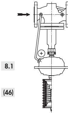
8.1 (46) Aukšto slėgio valdymo linija
