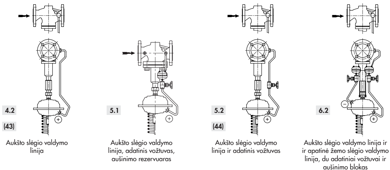
8.2 pav.: Montavimui paruoštos valdymo linijos 42-14 tipui, 42-18 tipui, 42-24 tipui, 42-28 tipui, skirtos montuoti srauto vamzdyje
