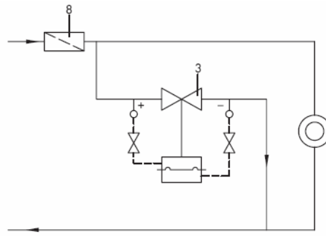
Nyomáskülönbség-szabályozás fűtő- vagy hűtőkészülék bypass vezetékében (nem távhő)
