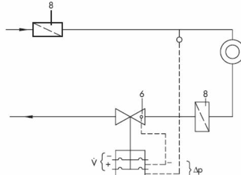
Kombinált mennyiség- és nyomáskülönbség-szabályozás fűtő- vagy hűtőkészülék visszatérő vezetékében
