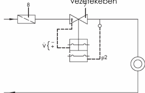
Kombinált mennyiség- és nyomáskülönbség-szabályozás
