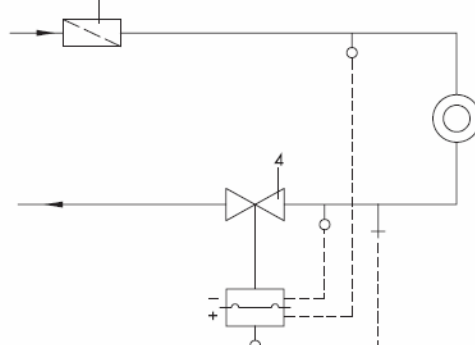
Nyomáskülönbség- és hőmérséklet-szabályozás
