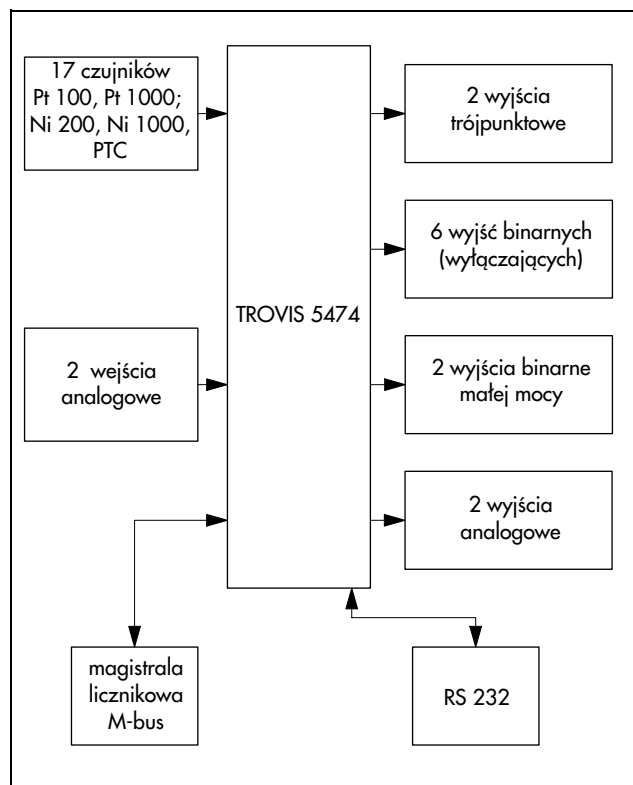
Rys. 2 · Wejścia i wyjścia regulatora
