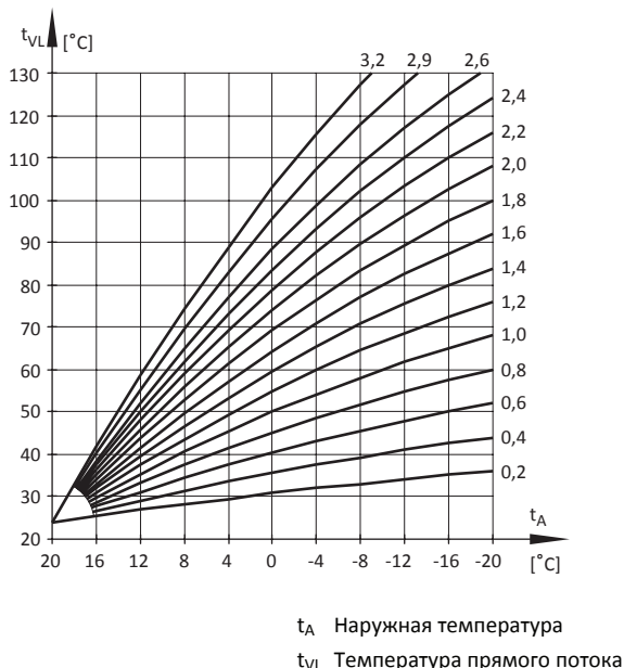
Рис. 2. · Характеристики отопления:
