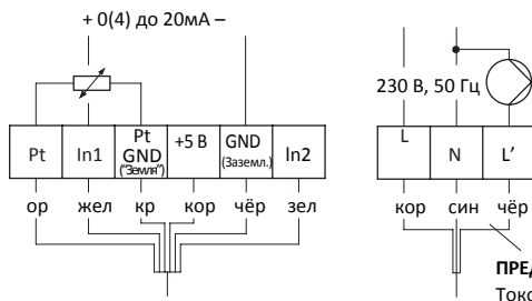
Схема с датчиком Pt 1000 и управление заданным значением посредством токового сигнала (Коммутационный выход L в качестве выхода для насоса)
