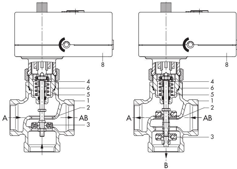
Bild 3: Wirkungsweise Typ 3226/5857 links: Mischventil, rechts: Verteilventil
