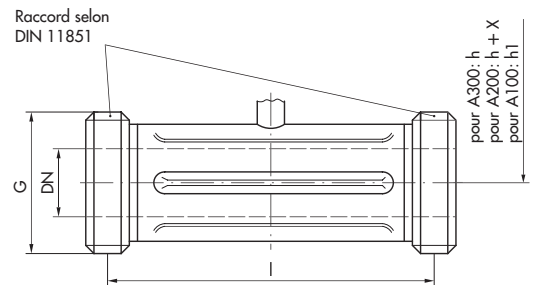
Fig. 12 · Dimensions en mm
