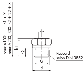
Fig. 8 · Dimensions en mm
