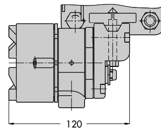
Montaje según NAMUR en tipo 4765 y tipo 3760
