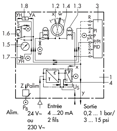
Régulateur indicateur pour le raccordement de transmetteurs 2 fils avec poste de commande type 3432-02 et poste de réduction d'air comprimé
