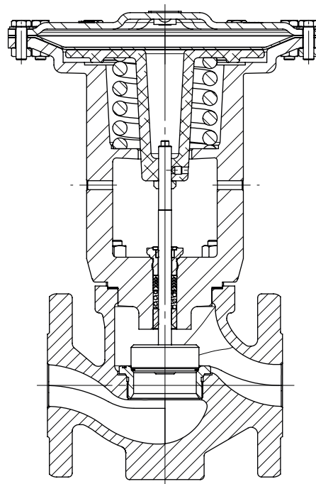
Fig. 5 : Vanne Tout ou Rien pneumatique type 3351 - Exécution „Ressort ouvre”
