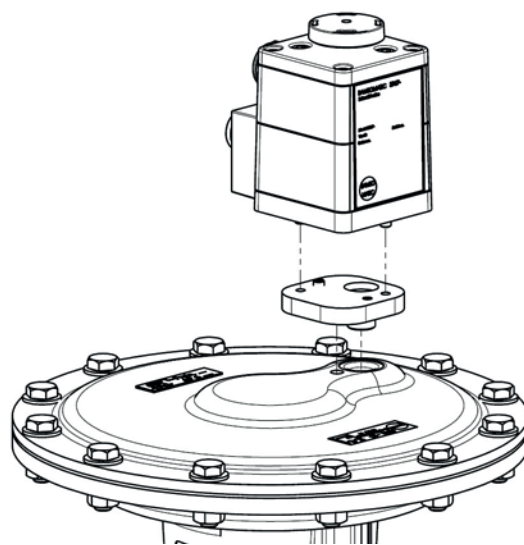
Fig. 6 : Plaque d'adaptation avec plan de pose NAMUR
