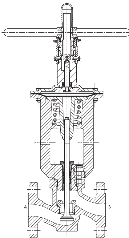
Fig. 4 : Vanne Tout ou Rien pneumatique type 3351 avec commande manuelle - Exécution „Ressort ferme”
