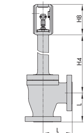
Typ 3256 mit Balg- oder Isolierteil
